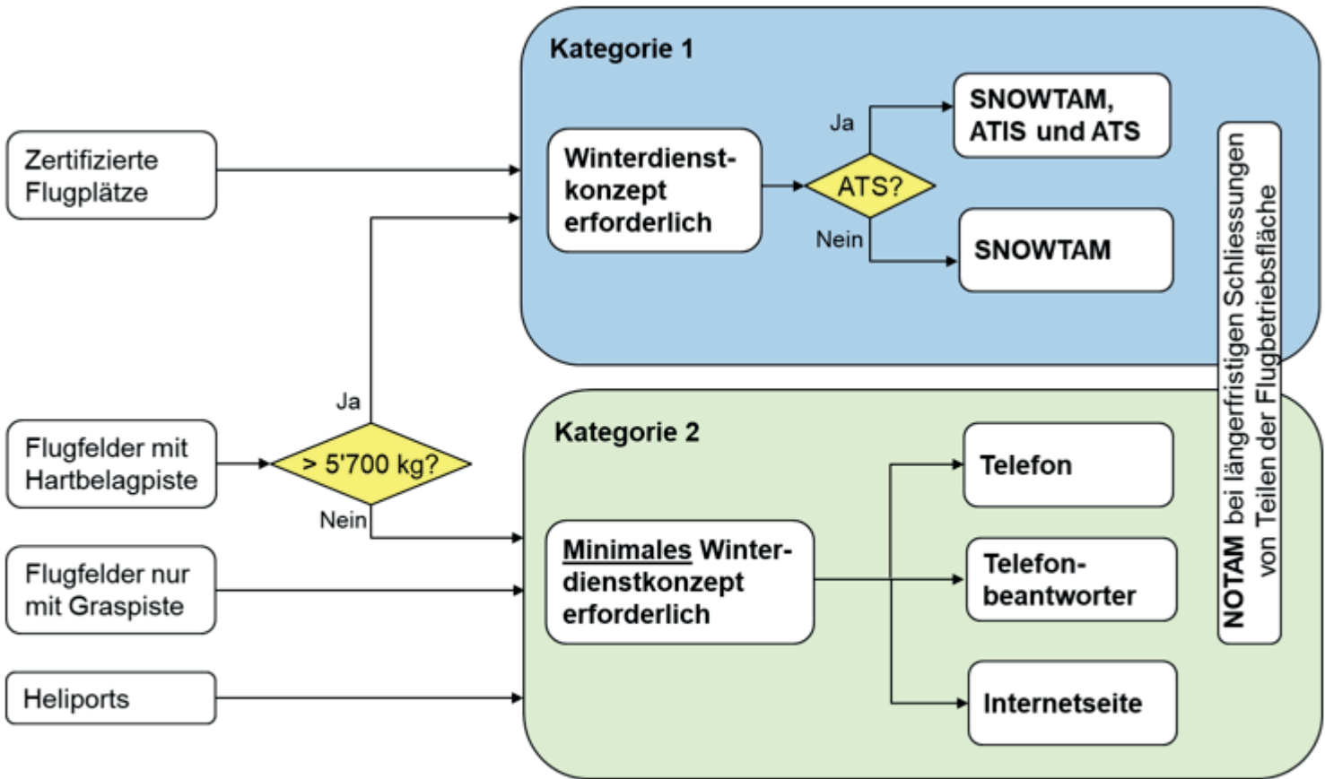
Abbildung 1: Kategorisierung der Flugplätze bei Winteroperationen nach Zertifizierungskriterien und Gewicht von Luftfahrzeugen
